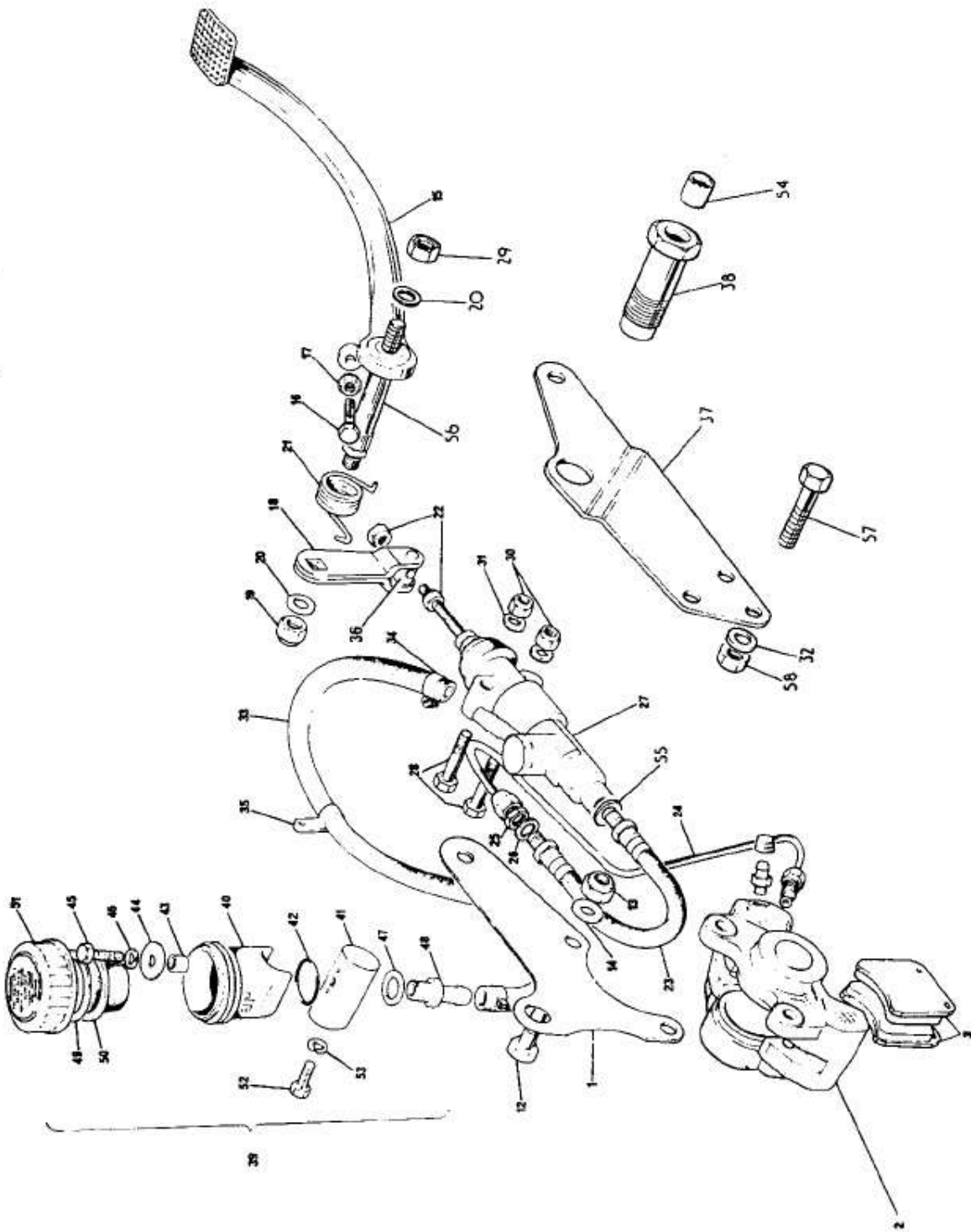
FIG. 25. REAR BRAKE
