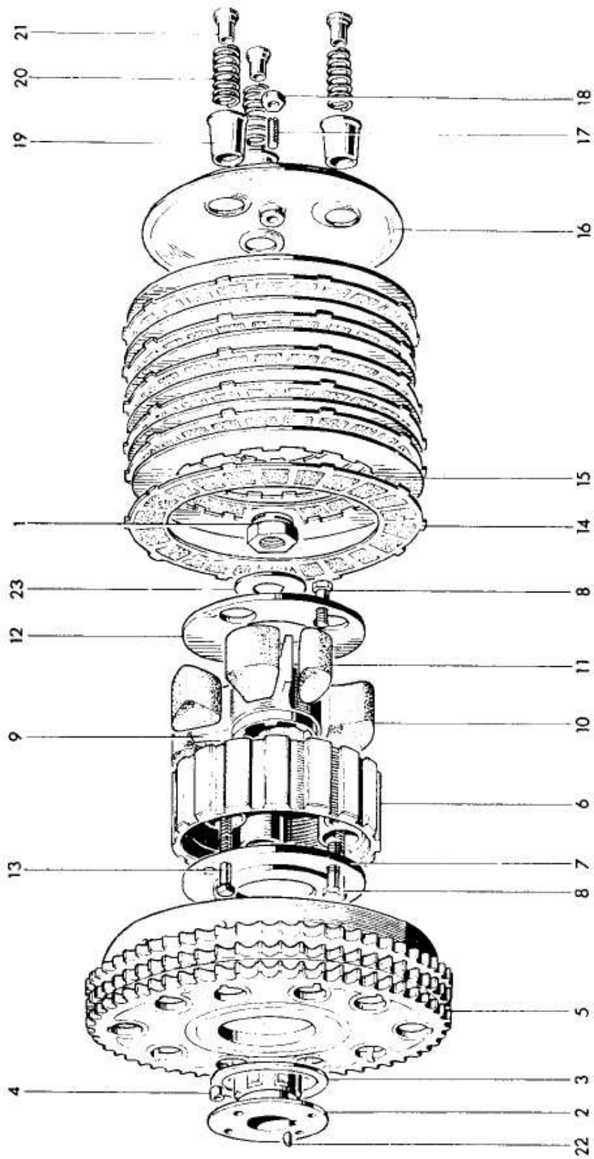
Fig. 14. CLUTCH
