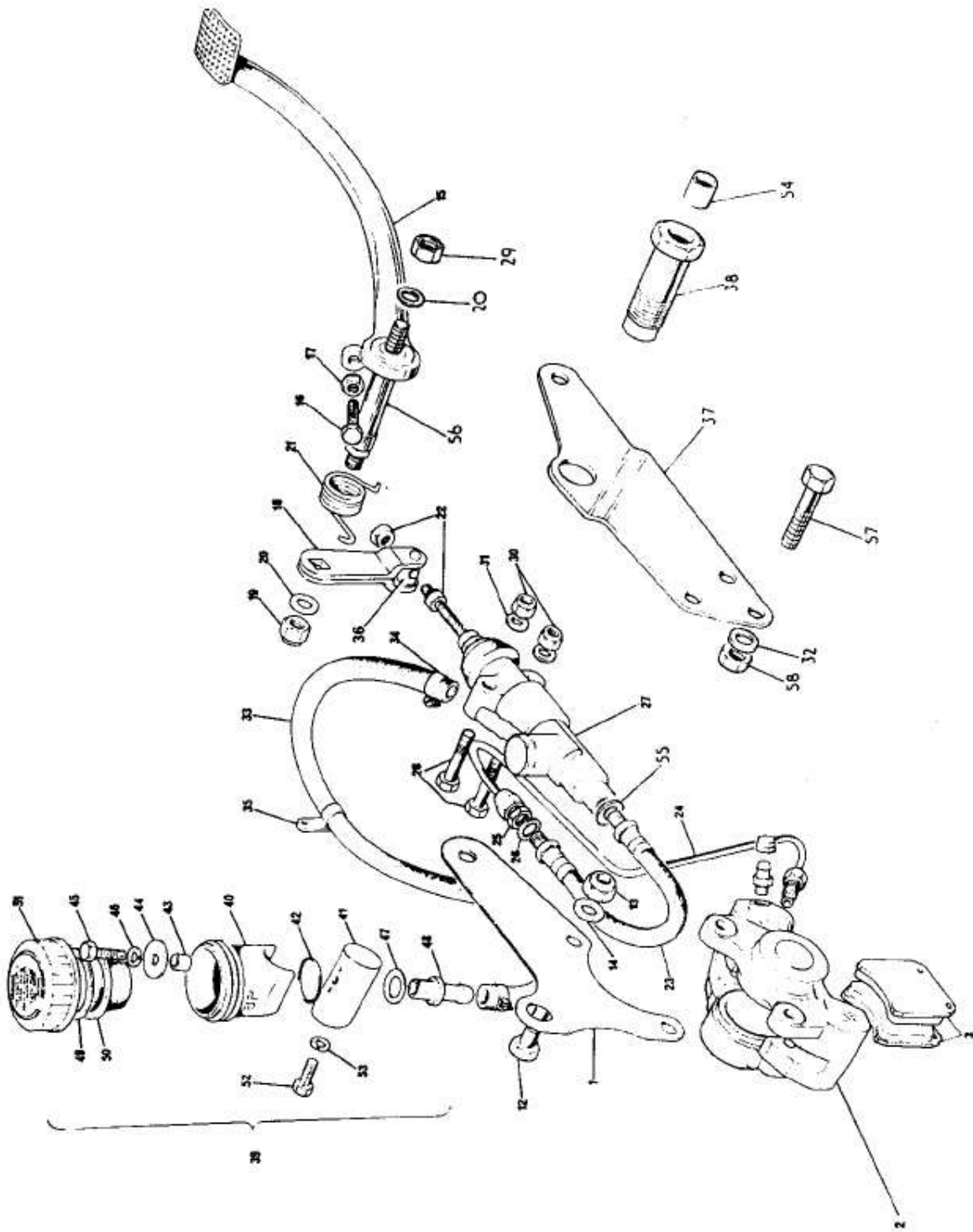
FIG. 25. REAR BRAKE
