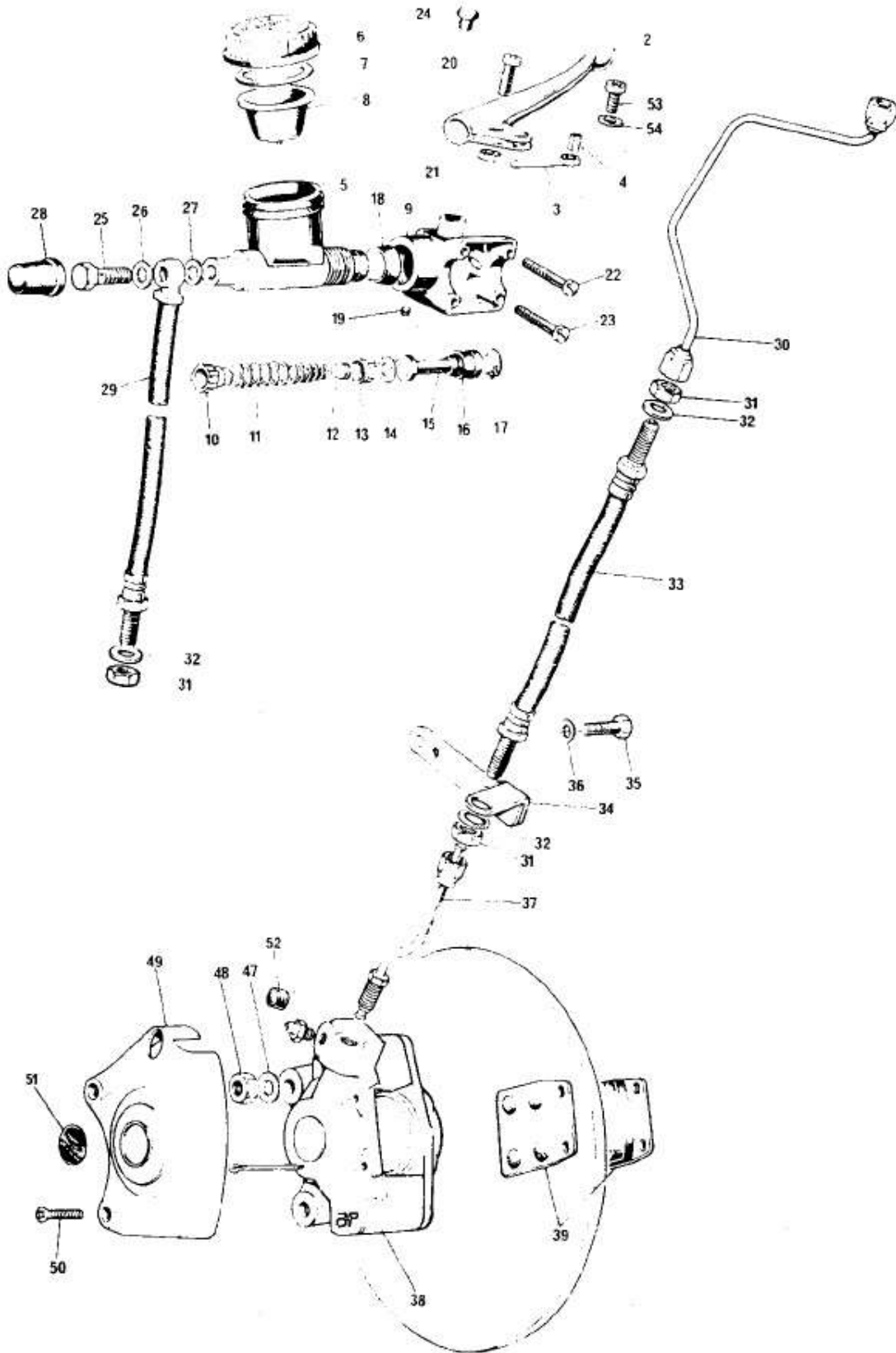
Fig. 23. FRONT BRAKE
