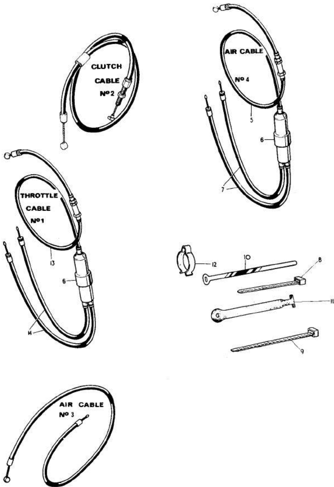
Fig. 30. CONTROL CABLES
