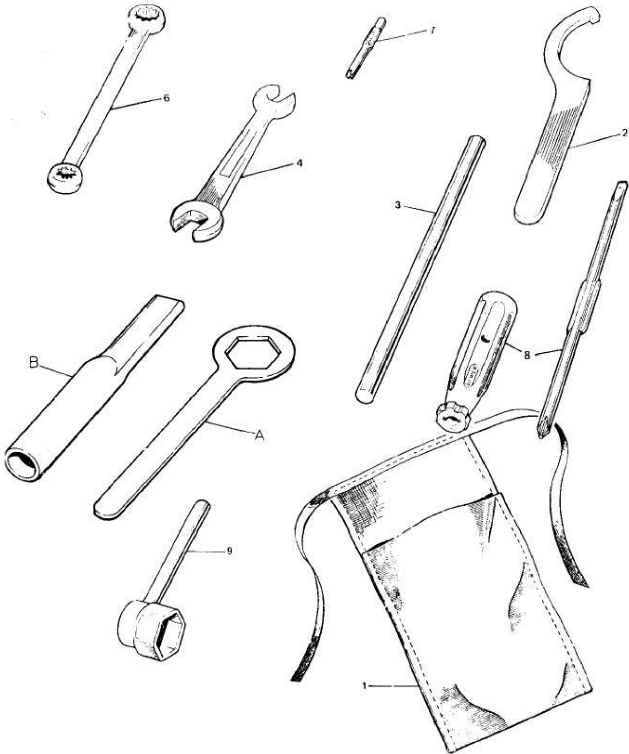
F.g. 31. TOOLKIT
