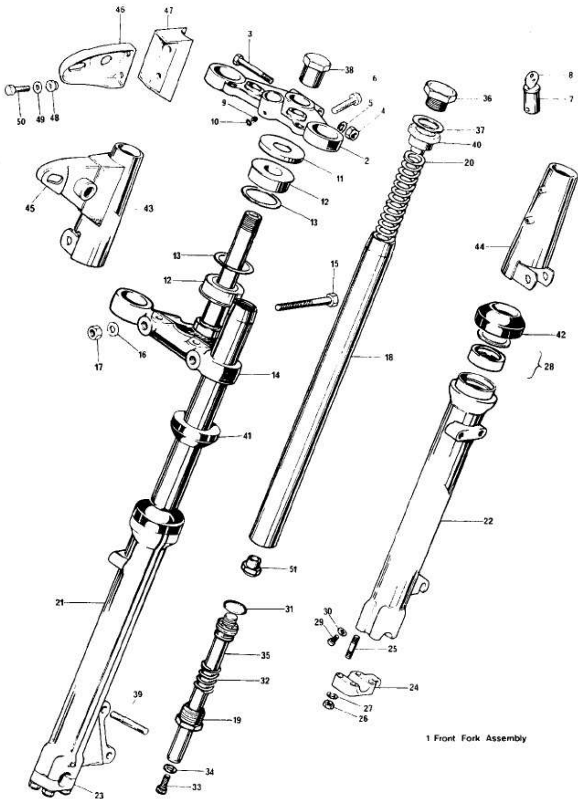
Fig. 20. TELESCOPIC FRONT FORK
