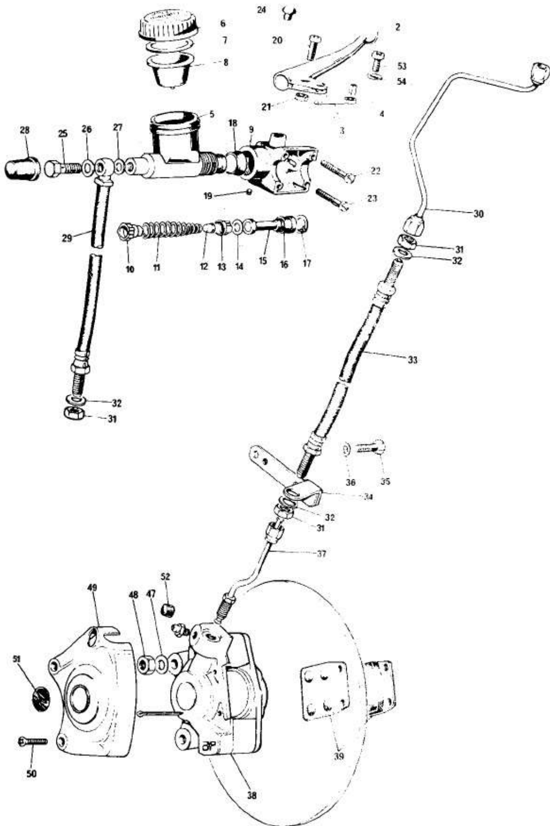
Fig. 23. FRONT BRAKE
